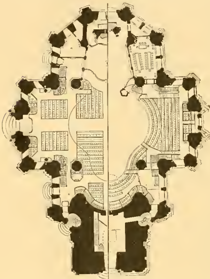
Fig. 144 Michaeliskirche zu Hamburg. Grundriss des Erd- und Obergeschosses.
